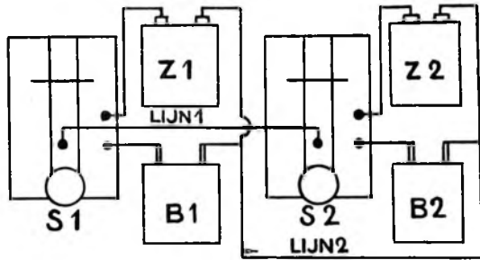
Fig. 6. Verbindingsschema voor twee sleutels en twee zoemers. Inplaats van Z1 en B1 en Z2 en B2 aan lijn 2 te verbinden kunnen deze ook aan een of andere aardverbinding bevestigd worden, b.v. de aanvoerbuis van de waterleiding.
