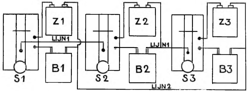
Fig. 7. Verbindingsschema voor drie sleutels en drie zoemers.
